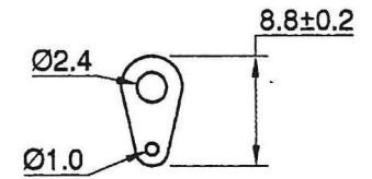
SOLDER LUG
